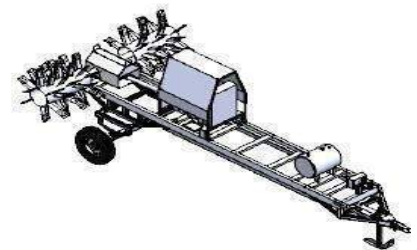
Aireador Auxiliar con motor Diesel Vista isométrica
